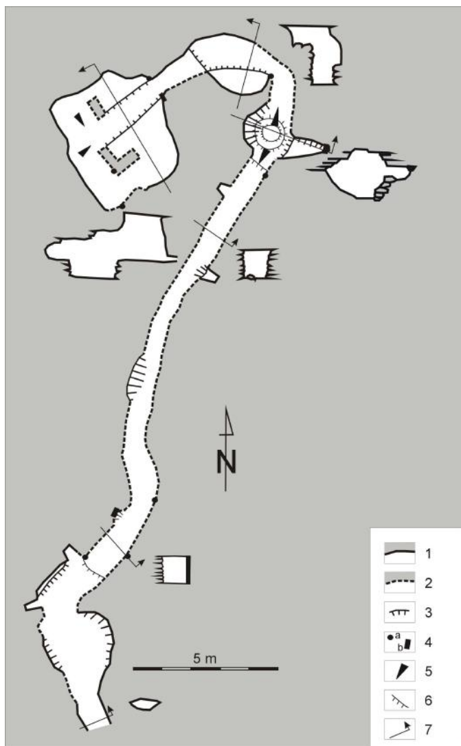
Ryc. 22. Plan i przekroje poprzeczne jednej z mniejszych sztolni w Potoku Senderkach (wg Urban, Młeczek 2011, zmodyfikowane). Objaśnienia oznaczeń (na planie): 1 – ściana skalna, 2 – ściana korytarza wykonana z bloków skalnych, 3 – skarpa luźnego materiału w ścianie lub przy dnie korytarza, 4 – elementy drewnianej obudowy: a – stempel, b – belka pozioma, 5 – nachylenie dna korytarza, 6 – nachylony element stropu korytarza, 7 – przekrój poprzeczny.
