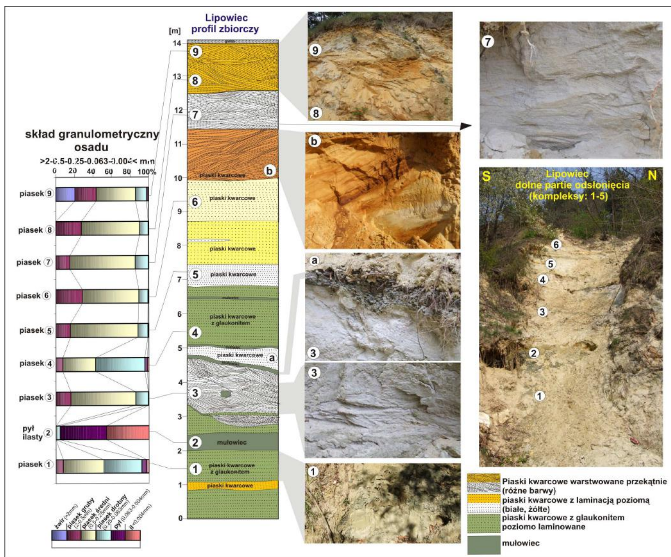
Ryc. 3. Zbiorczy profil utworów piaszczystych miocenu w Lipowcu. Fot. W. Margielewski.
