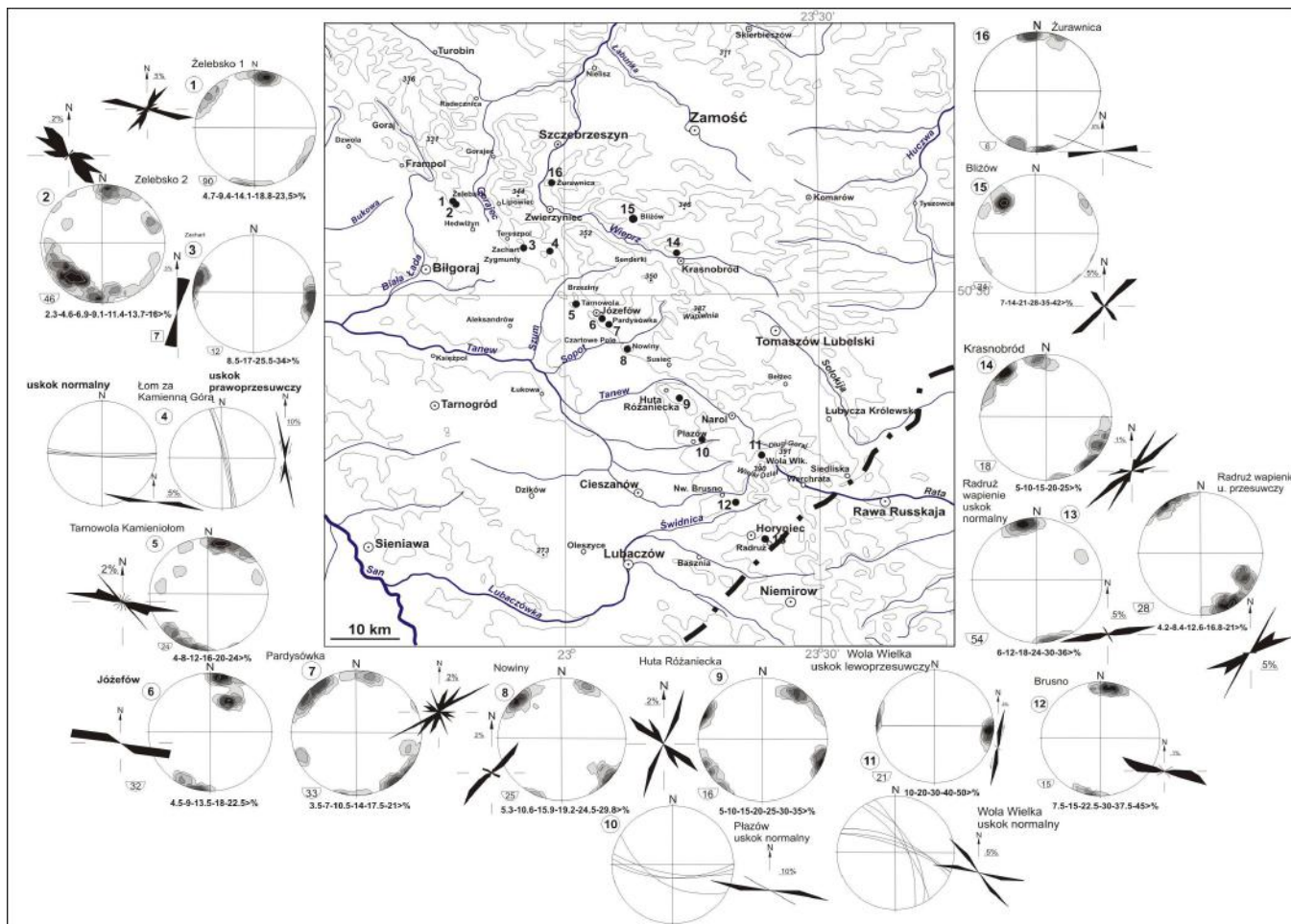
Ryc. 5. Położenie płaszczyzn uskoków w obrębie skał Roztocza, na diagramach kierunkowych i konturowych (projekcja równopowierzchniowa biegunów na dolną półkulę (obok diagramów zaznaczono ilość pomiarów i wartość poziomic) Część płaszczyzn uskoków jest prezentowana na diagramach kołowych (projekcja na dolną półkulę) (Jankowski, Margielewski 2014b).
