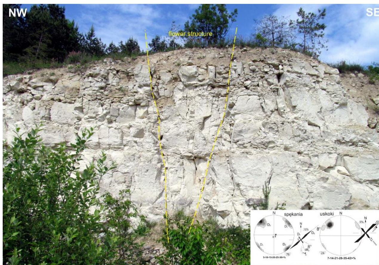
Ryc. 19. Odsłonięcie opok kredowych w kamieniołomie w Bliżowie. W centralnej części ściany widoczna struktura kwiatowa związana z uskokiem prawoprzesuwczym. Poniżej diagramy spękań i uskoków (wg: Jankowski, Margielewski 2014). Objaśnienia do diagramów spękań jak na ryc. 10. Fot. W. Margielewski.
