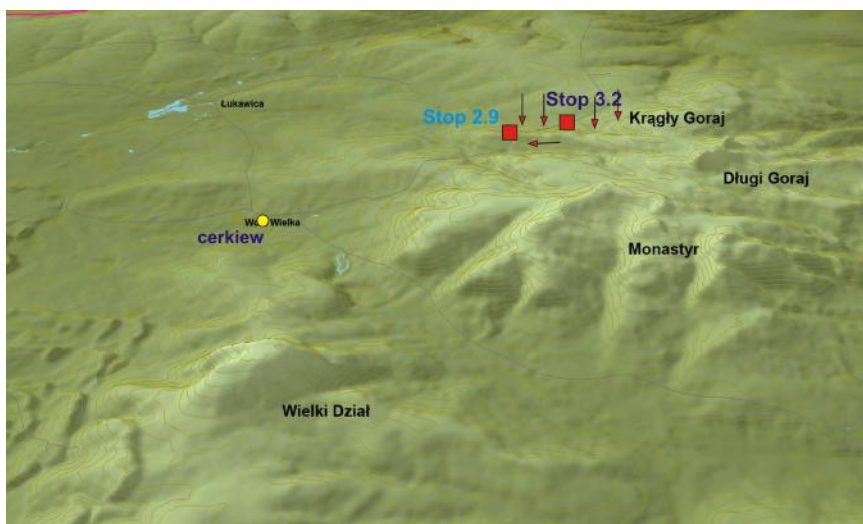
Ryc. 43. Miejsce występowania fragmentów skrzemieniałego drewna (zaznaczono strzałkami) na polach ornym otaczających Kragły Goraj.
