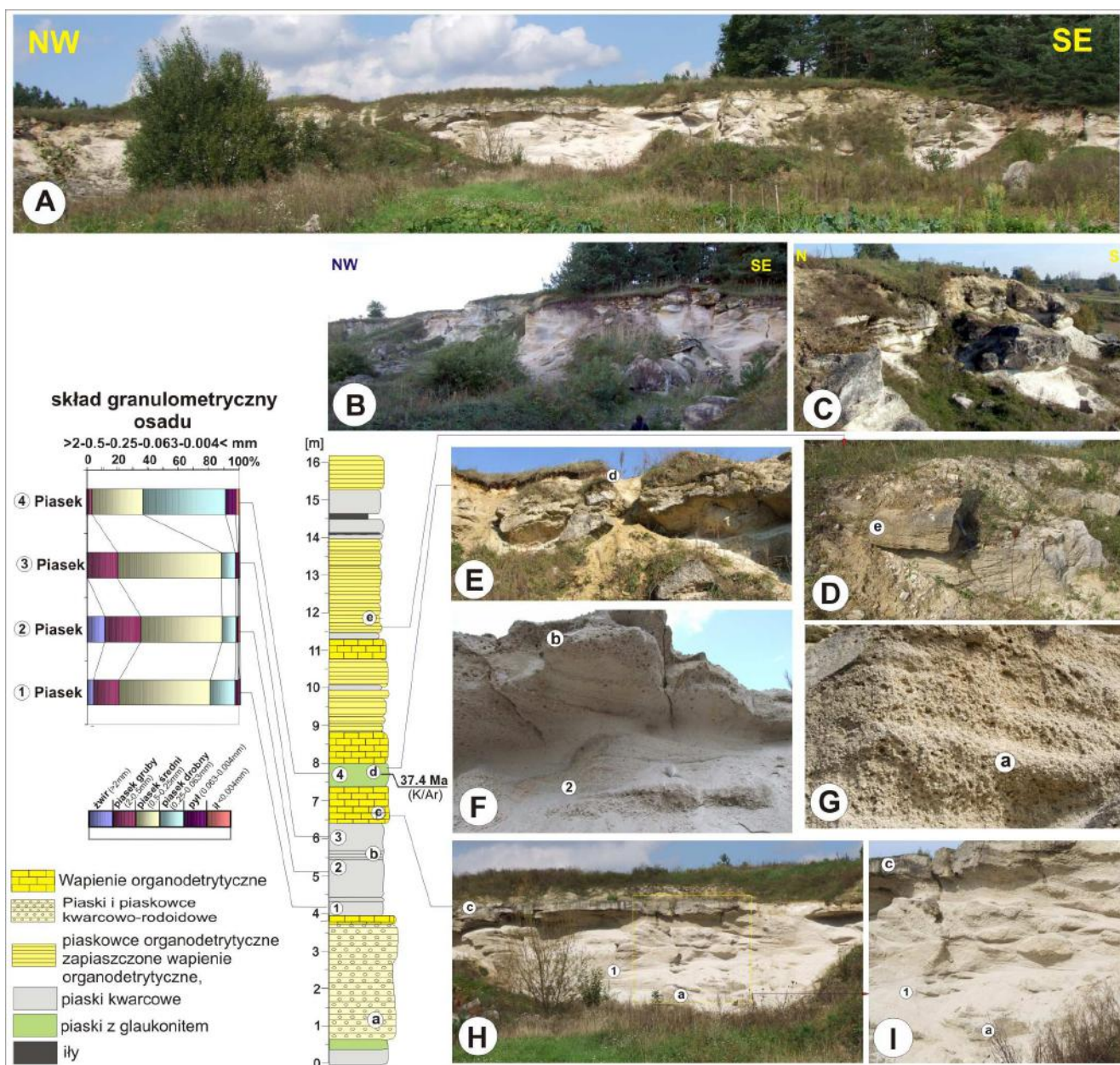
Ryc. 35. Zbiorczy profil utworów miocenu odsłaniających się w Hucie Różanieckiej (profil wg Wysockiej 2006 a, b). Fot. W. Margielewski.
