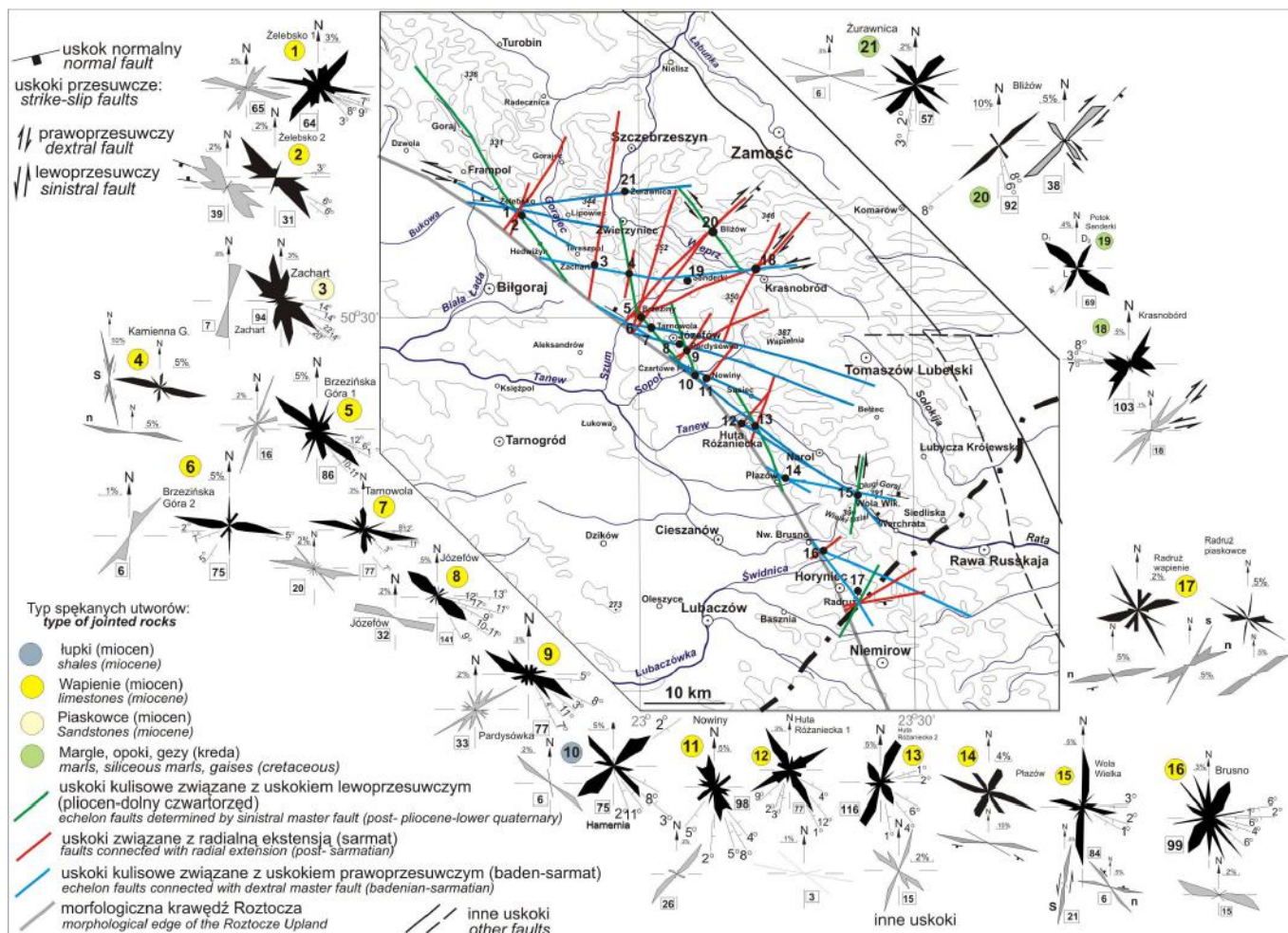
Ryc. 4. Przebieg nieciągłości tektonicznych (uskoki, spękania) w obrębie skał Roztocza, na diagramach kierunkowych: czarne – spękania, z położeniem warstw, szare: uskoki. W kwadratach podano ilość pomiarów (za: Jankowski, Margielewski 2014b).
