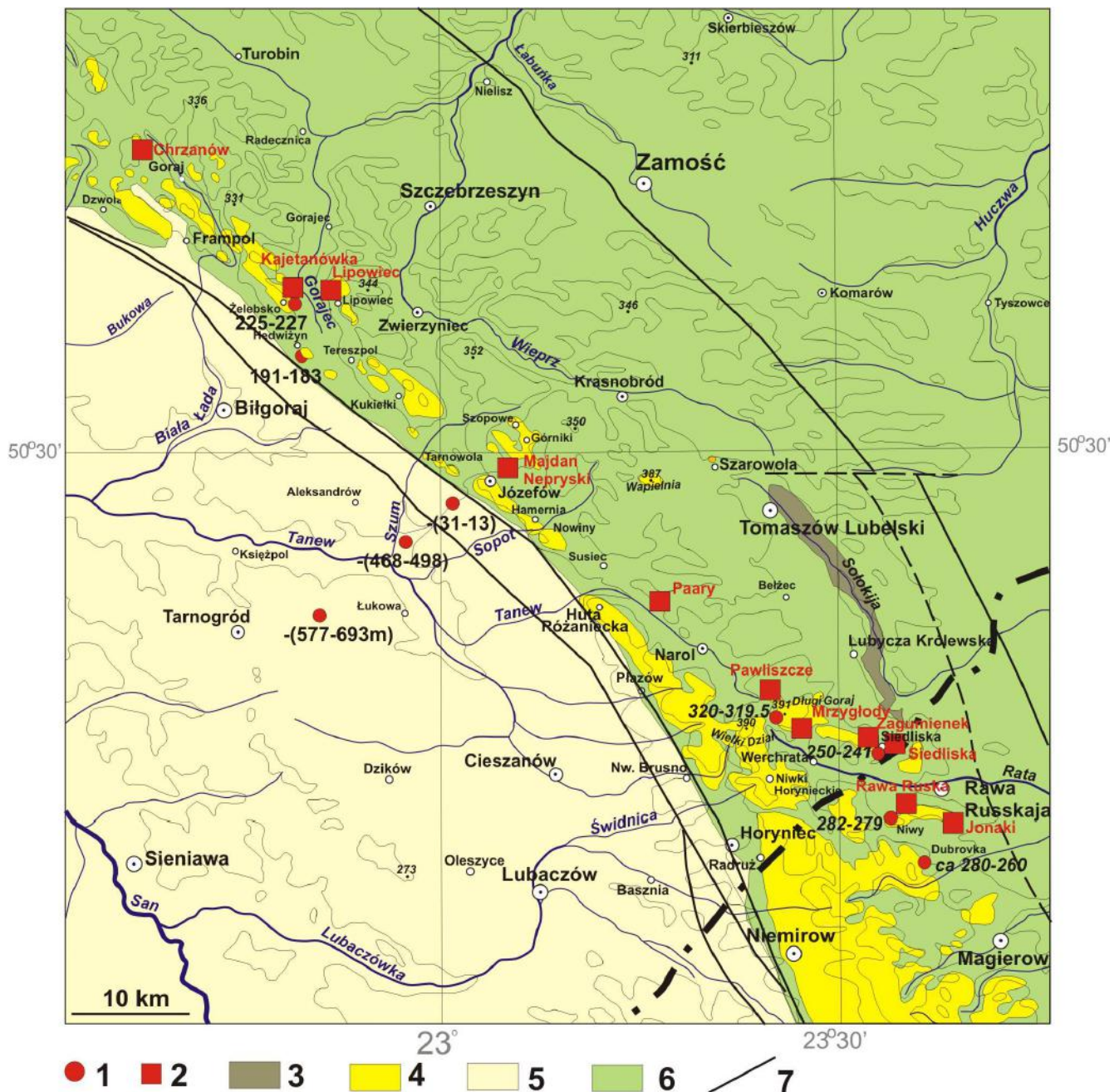
Ryc. 2. Występowanie fosylnego drewna na Roztoczu i w brzeżnej części zapadliska przedkarpacciego, na tle uproszczonej mapy geologicznej regionu. 1 – poziomy lignitów formacji z Trzysznicy nawiercone w podłożu na różnych głębokościach (zakres głębokości podany w wysokościach bezwzględnych); 2 – powierzchniowe nagromadzenia zsylikowanego drewna (wg Krapiec i in., 2011); 3 – utwory eocenu; 4 – utwory miocenu Roztocza (piaski, piaskowce, wapień); 5 – osady zapadliska przedkarpacciego; 6 – krzemionkowo-wapienne utwory kredowe, 7 – dyslokacje (geologia wg. Buraczyński 2002, Wysocka 2006, Oszczytko 2006).
