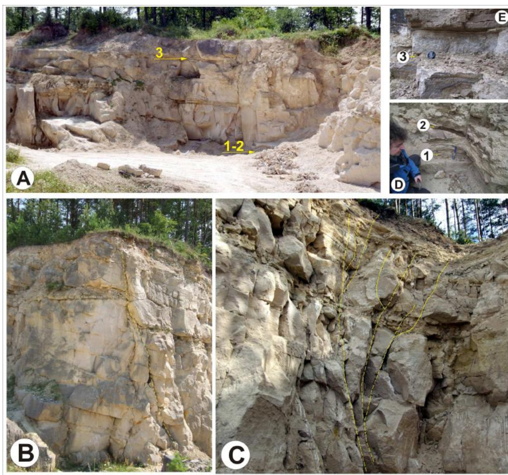
Ryc. 25. Kamieniołom w Józefowie, część wschodnia wyrobisk. W obrębie wapieni organodetrytycznych widoczne są poziomy utworów pylastych (Fot. A – poziomy 1-3; Fot. D-E). Skały pocięte są spękaniami oraz uskokami: normalnymi zrzutowymi (fot. B) i przesuwczymi, tworzącymi tu struktury kwiatowe (Fot. C). Fot. W. Margielewski.
