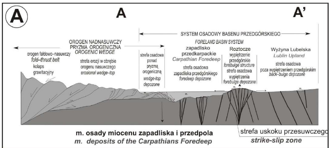
Ryc. 10. Pozycja Roztocza (jako struktury forebulge ) w systemie depozycyjnym zapadliska przedkarpackiego. Interakcja pomiędzy formowaniem struktur kwiatowych stowarzyszonych z uskokami przesuwczymi, a formowaniem wypiętrzenia przedgórskiego ( forebulge ) związanego z nasuwaniem się górotworu Karpat na przedpole, dzielącego basen na poszczególne strefy osadowe (wg schematu: DeCelles, Giles 1996 i Krzywca 2006, uzupełniony i zmieniony :Jankowski, Margielewski, 2014b). Zasięg utworów sarmatu wg Gąsiewicz i in. 2004.
