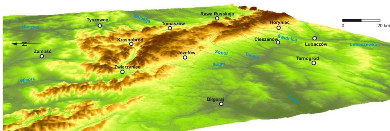
Ryc. 1. Położenie Roztocza. Na rzucie ortogonalnym SRTM zwraca uwagę skośny przebieg linii nie rozwiniętych form rzeźby Roztocza (dolin, grzbietów) do kierunku strefy krawędziowej
