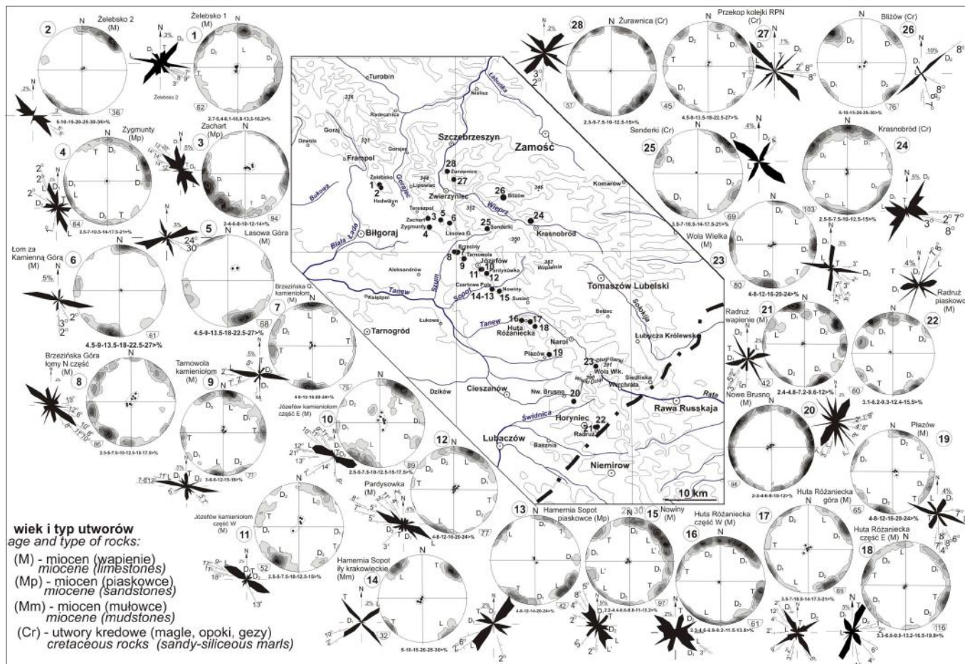
Ryc. 6. Położenie płaszczyzn spękań w obrębie skał Roztocza, na diagramach kierunkowych i konturowych (objaśnienia – zob. ryc. 5); Przestrzenne położenie warstw na diagramach punktowych (projekcja na dolną półkulę) (Janowski, Margielewski, 2014b).
