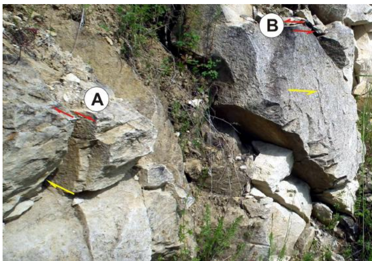
Ryc. 20. Bliżów, uskoki przesuwowe w opokach kredowych: A – prawoprzesuwowy ( dextral ), B – lewoprzesuwowy ( sinistral ). Żółta strzałka wskazuje kierunek ruchu bloku przyległego. Fot. W. Margielewski.
