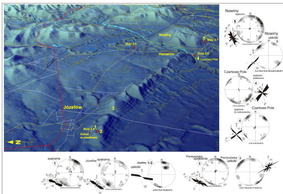
Ryc. 24. Charakterystyczny wał strefy krawędziowej Roztocza, pomiędzy Józefowem i Nowinami (numeryczny model terenu), z kamieniołomami w Józefowie (Stop 2.4); Pardysówce (p. 3), przełomem Sopotu przez strefę krawędziową (Stop 2.6) i wyniesionym masywem Nowin z Kamieniołomem w Błudku (Stop 2.7). Spęknięcia i uskoki dla skał poszczególnych stanowisk – na diagramach konturowych i kierunkowych (objaśnienia zob. ryc. 10). Czerwonym kółkiem zaznaczono kirkut w Józefowie
