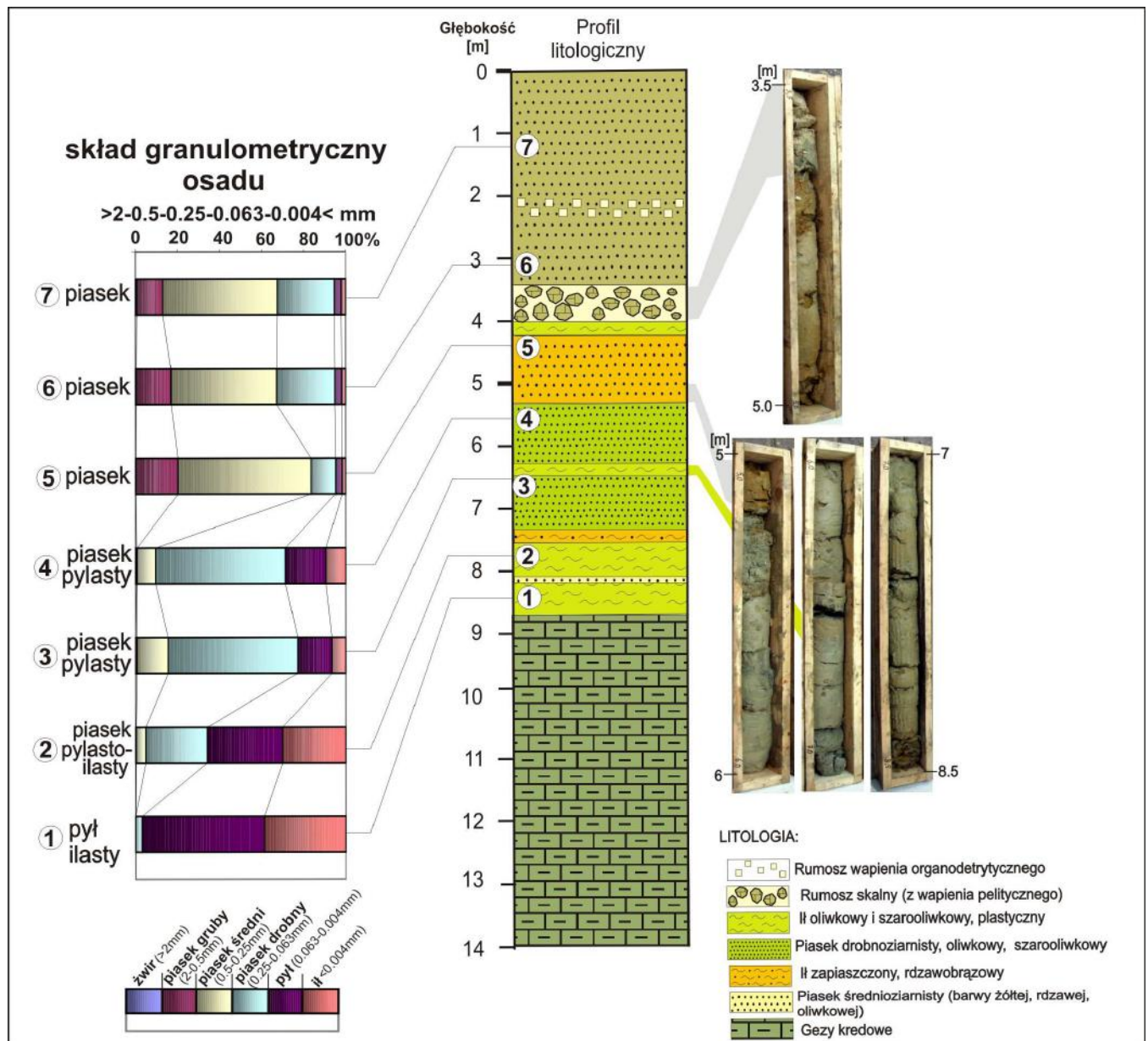
Ryc. 4. Profil wiercenia utworów piaszczystych w Lipowcu (wg Krapiec i in. 2011).
