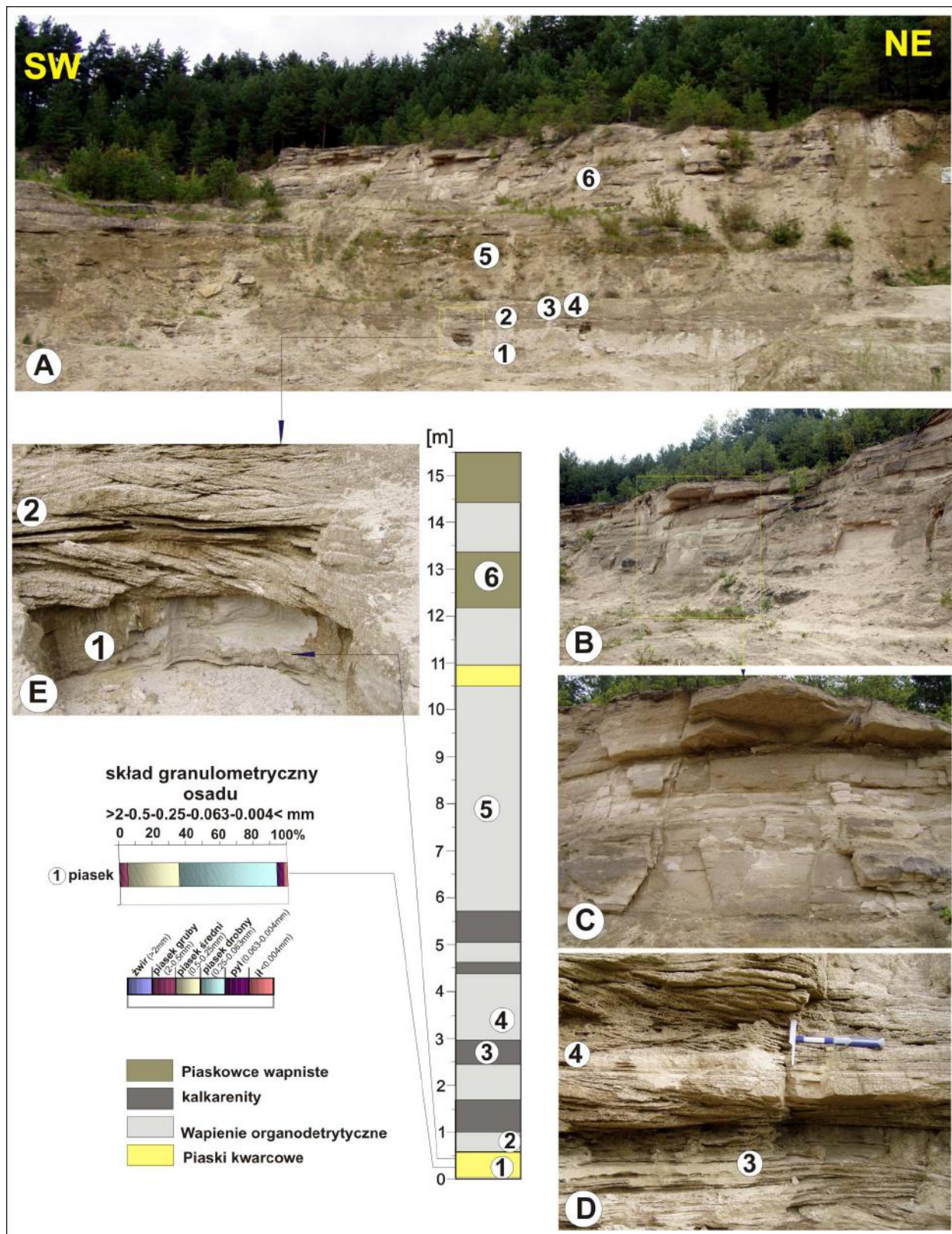
Ryc. 33. Odślonienie utworów miocenu w kamieniołomie w Błudku-Nowinach. Profil litologiczny wg Wysockiej 2002, uproszczony. Fot. L. Jankowski, W. Margielewski.
