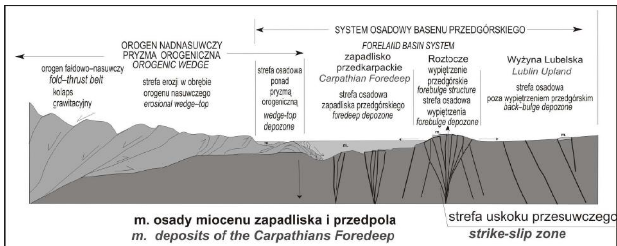
Ryc. 34. Pozycja Roztocza (jako struktury forebulge ) w systemie depozycyjnym zapadliska przedkarpackiego, dzielącego basen zapadliska na poszczególne strefy osadowe (Jankowski, Margielewski 2014, wg. schematu: DeCelles, Giles 1996 i Krzywca 2006).
