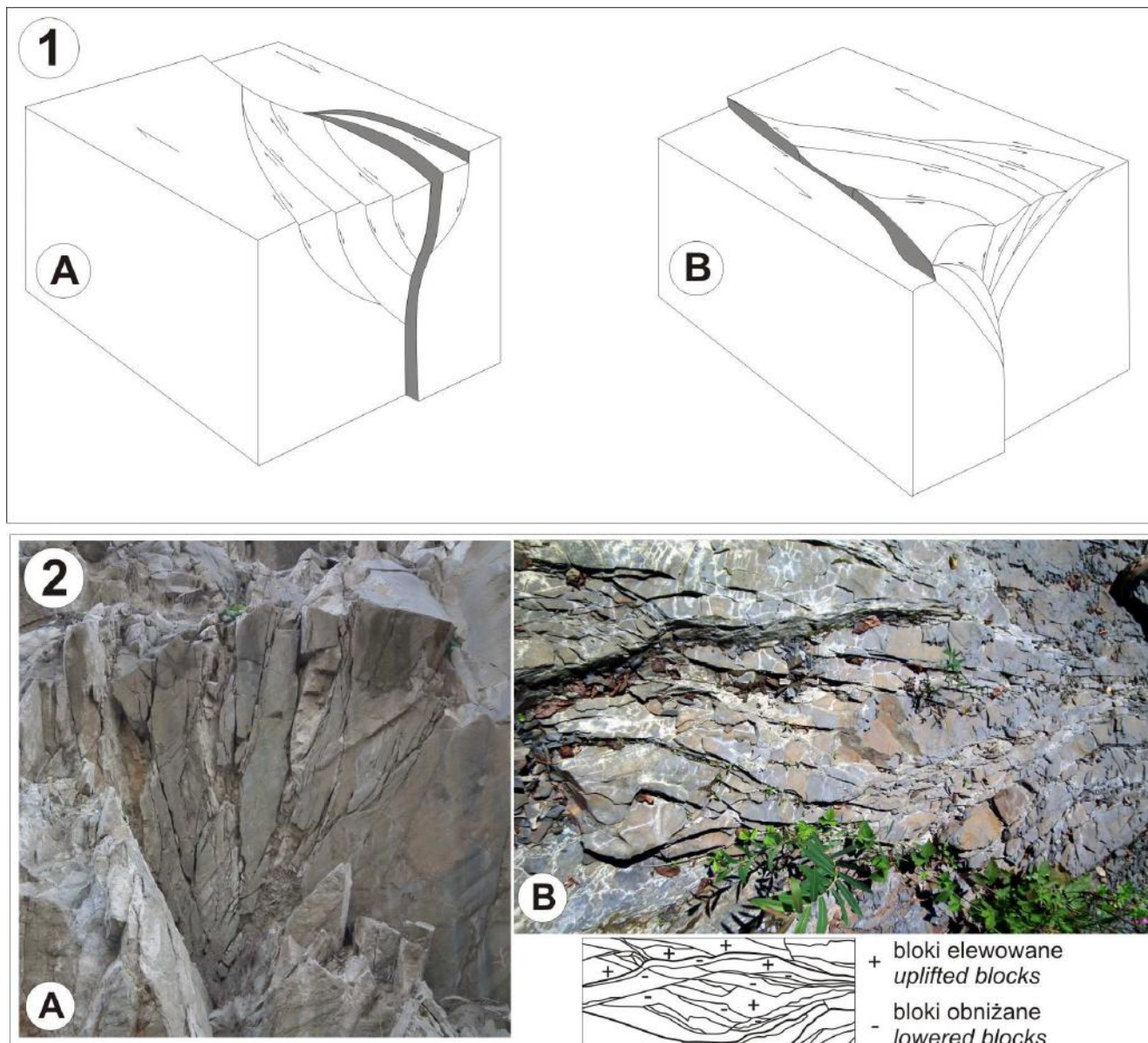
Ryc. 8. Struktura kwiatowa ( flower structure ): model ilustrujący formowanie się wyniesionej struktury Roztocza. 1 – model tworzenia struktur kwiatowych stowarzyszonych z uskokiem przesuwczym: A – struktura negatywna (tulipanowa); B – struktura pozytywna (palmowa) (wg Dadleza i Jaroszewskiego 1994). 2 – przykład struktur kwiatowych w mezoskali: A – przekrój poprzeczny przez strukturę kwiatową formowaną przez uskoki prawoprzesuwcze (piaskowce magurskie, kamieniołom w Wierchomli, Beskid Sądecki); B – przykład górnej powierzchni struktury kwiatowej z elementami obniżanymi i elewowanymi (margle podcergowskie, Lipowica, Beskid Niski, koryto Jasiołki) (Jankowski, Margielewski 2014b).
