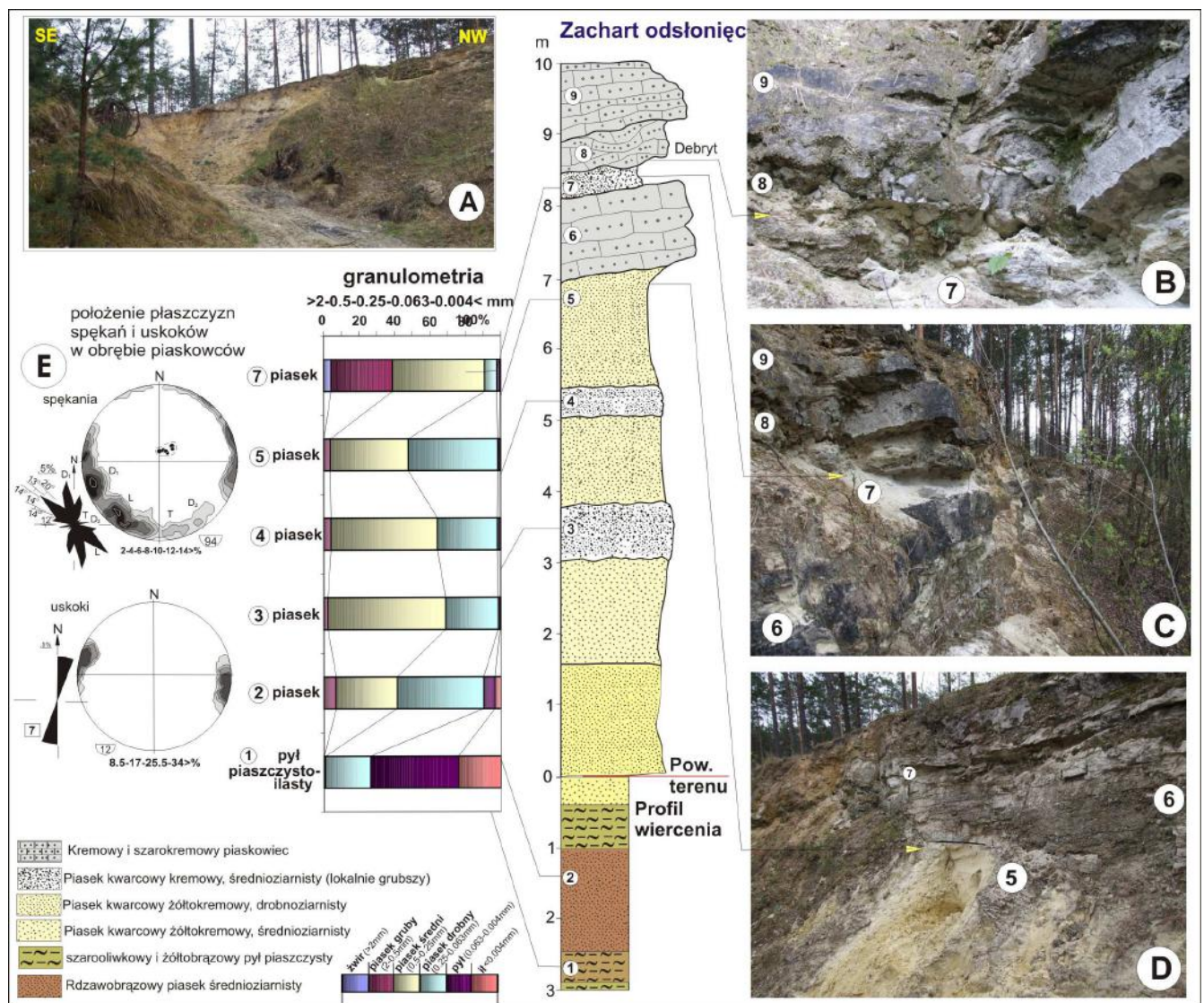
Ryc. 10. Profil odsłonięcia i wiercenia utworów miocenu w Zacharcie. Położenie płaszczyzn spękań i uskokuw (w piaskowcach) na diagramie konturowym (projekcja równopowierzchniowa biegunów na dolną półkulę) i kierunkowym (za: Jankowski, Margielewski 2014). Fot. W. Margielewski.
