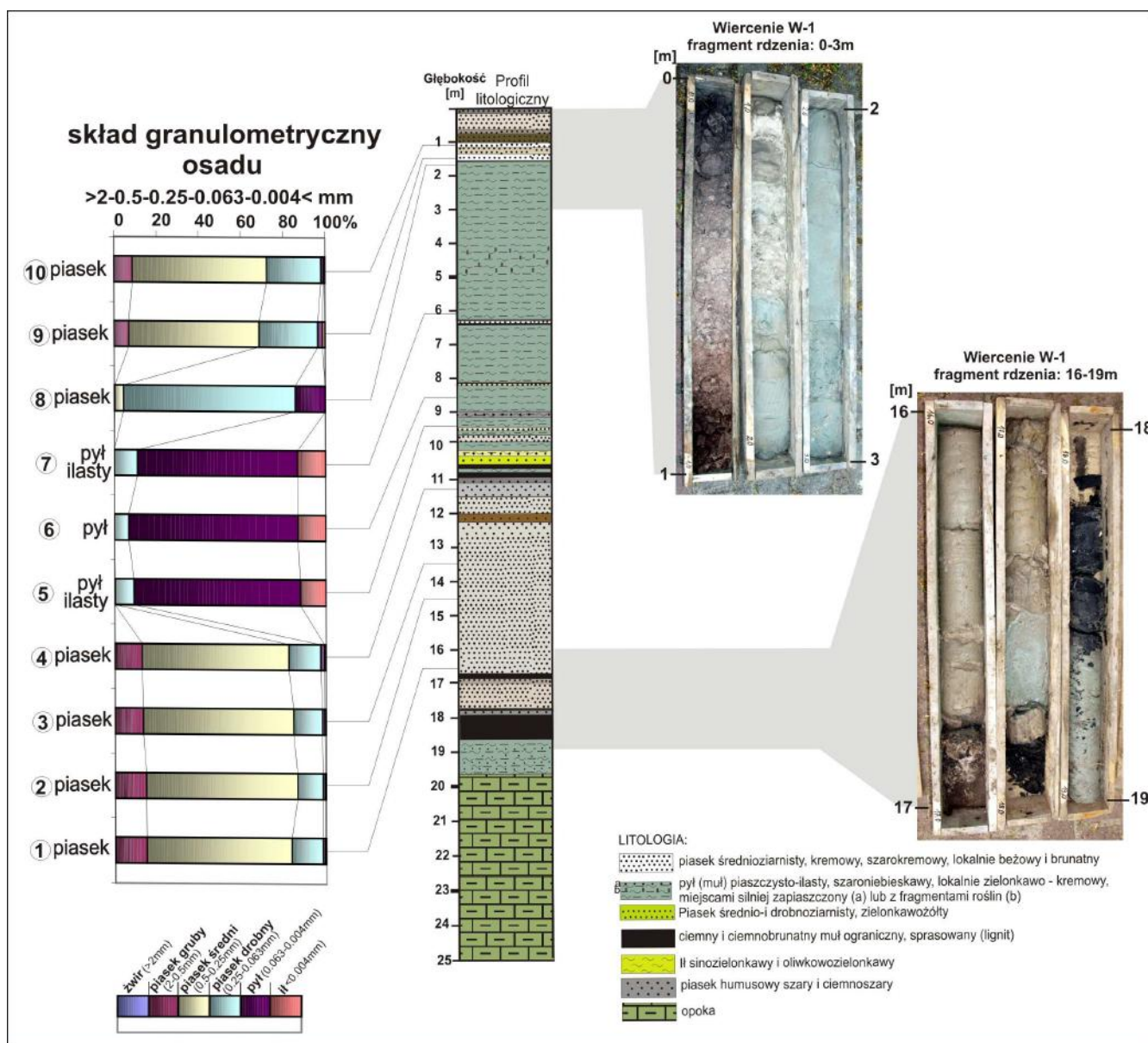
Ryc. 48. Profil wiercenia w Siedliskach z nawierconą sekwencją burowęgla. Z prawej rdzenie z widocznymi poziomami lignitów (wg Krąpiec i in. 2011) (fot. W. Margielewski).
