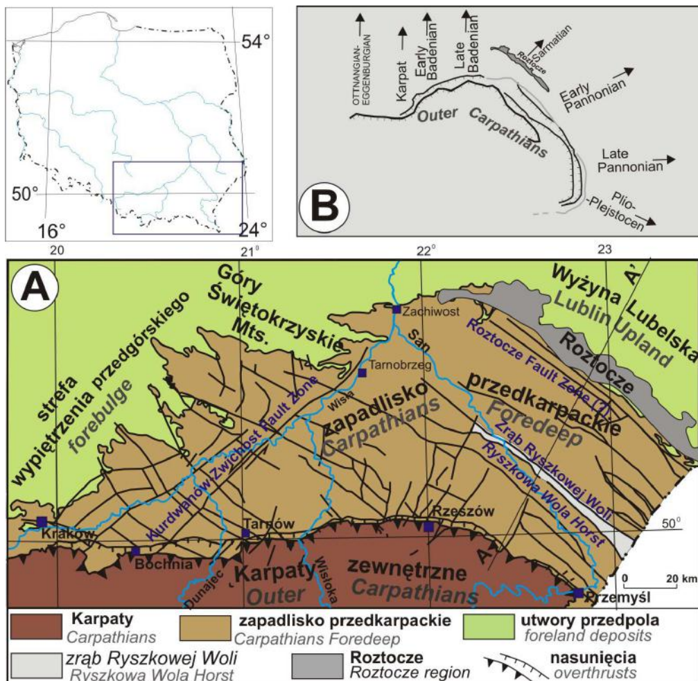
Ryc. 9. Relacja przestrzenna Karpat i zapadliska przedkarpackiego z wyniesioną strukturą Rostocza, do struktur przedpola (A) (za Oszczypko 2006). Uskoki obrzeżające zapadlisko i pozycja zrębu Ryszkowej Woli, za: Rauch 2009). Powyżej (B) zmiany kierunku nasuwania Karpat zewnętrznych w czasie (wg Royden, Baldi 1988)
