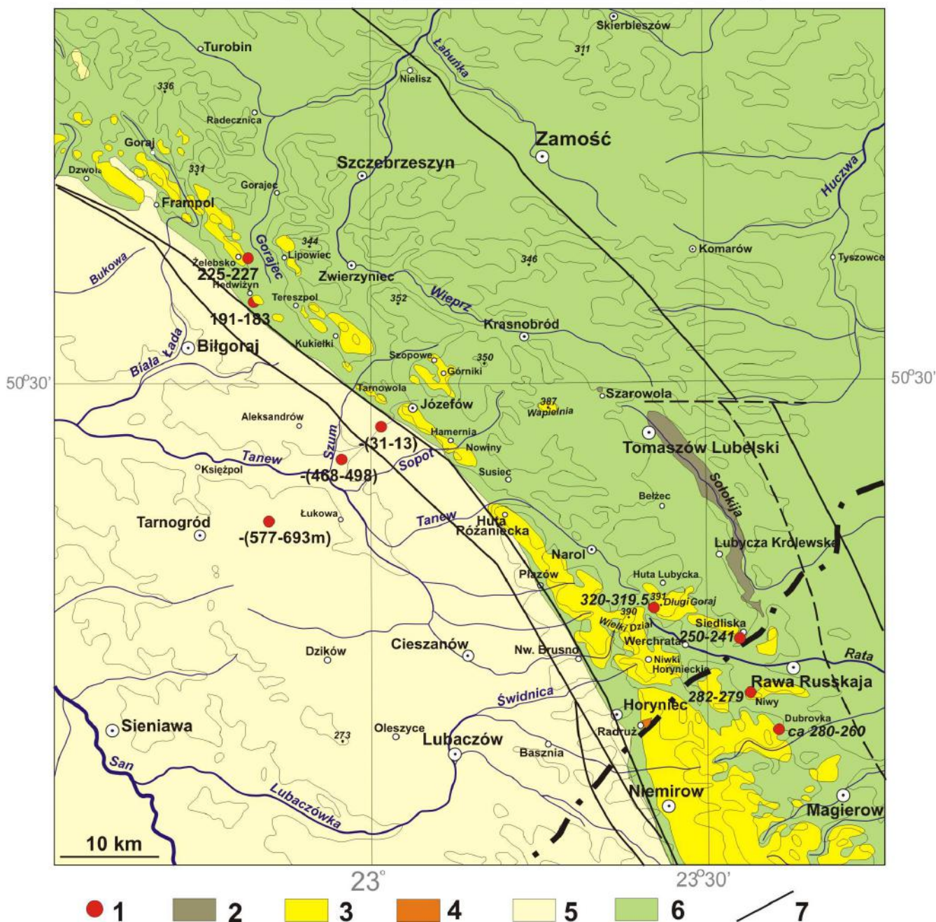
Ryc. 2. Uproszczona mapa geologiczna Rostocza Środkowego i Wschodniego, z zaznaczonym zróżnicowaniem występowania poziomu burowęgla (piętro karpatu) (mapa wg kompilacji Buraczyńskiego red. 2002; Wysockiej, 2006, zmieniona: Jankowski, Margielewski, 2014b). Objasnienia sygnatur: 1 – występowanie poziomu burowęgla na Rostocz i w zapadlisku (z podaniem w metrach wysokości bezwzględnej w stosunku do poziomu morza); 2 – utwory eocenu na Rostocz (Buraczyński red. 2002); 3 – miocénskie utwory piaszczyste i węglanowe (nierozdzielone); 4 – wapnienie z Radruża; 5 – utwory miocenu zapadliska przedkarpackiego; 6 – utwory węglanowo-krzemionkowe wieku kredowego; 7 – strefy dyslokacyjne obramowujące Rostocze wg: Buraczyński red. 2002; Oszczypko 2006, Wysocka 2006).
