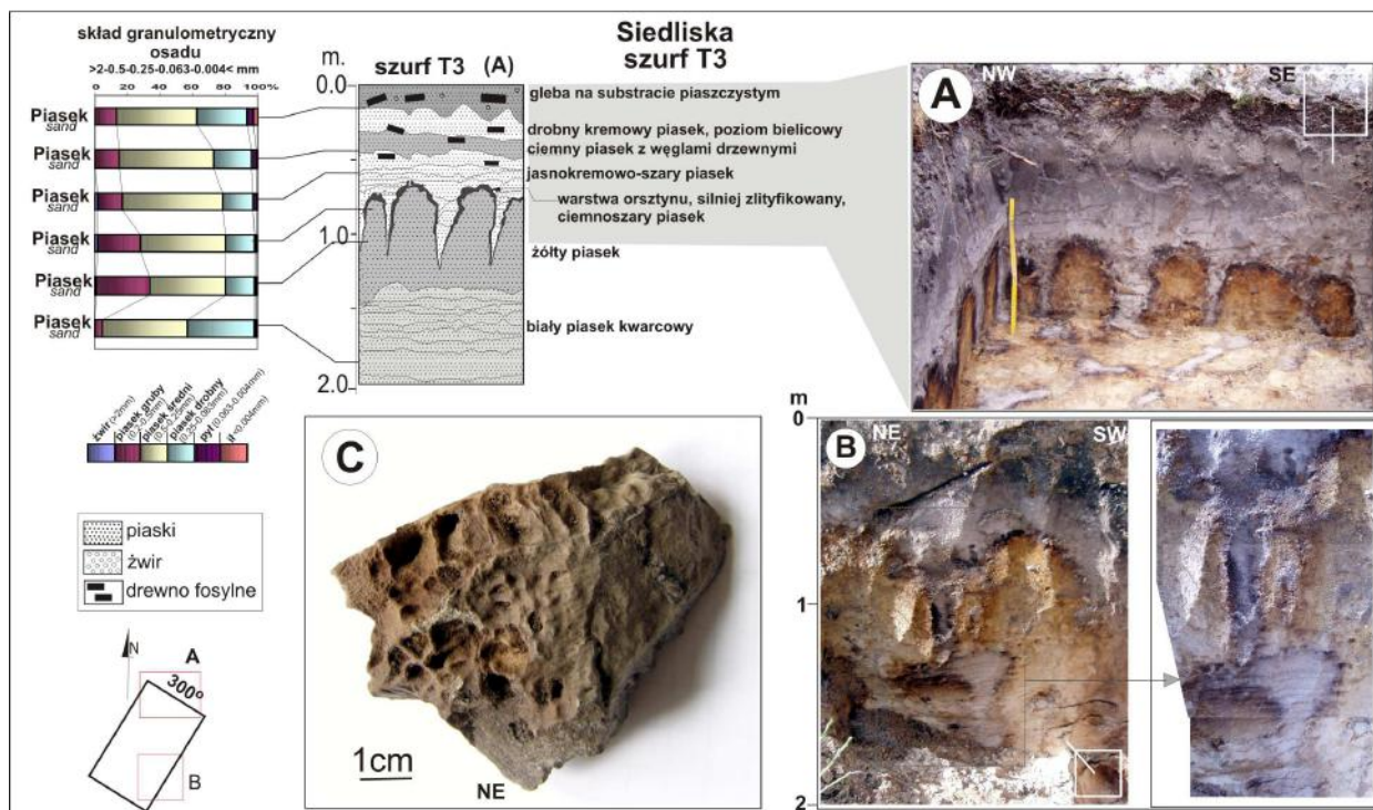
Ryc. 50. Profil utworów rzecznych terasy nadzalewowej Prutnika z charakterystycznymi klinami mrozowymi, wzbogaconych w fosylia. Siedliska, w pobliżu granicy Państwa (wg. Krąpiec i in., 2007). Fot. W. Margielewski.
