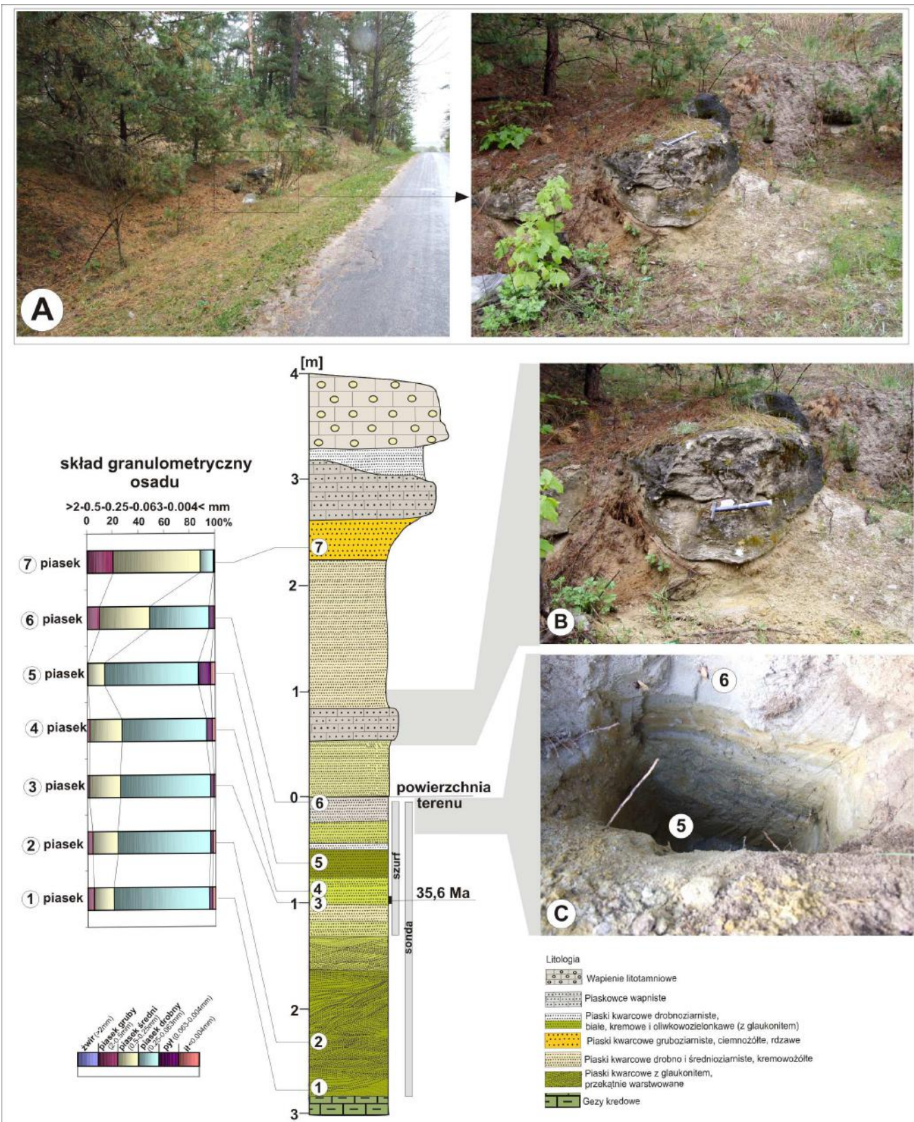
Ryc. 37. Profil utworów miocenu w Hucie Lubyckiej-Pawliszczach (Krapiec i in. 2011, por. także Józefkowicz 1976). Fot. W. Margielewski.
