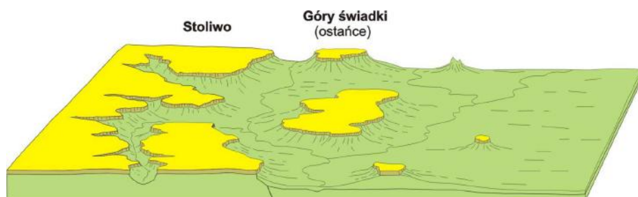
Ryc. 14. Schemat powstawania ostańców denudacyjnych (tzw. gór-świadków) (wg Migoń 2006), w układzie litologicznym charakterystycznym dla strefy krawędziowej Roztocza.
